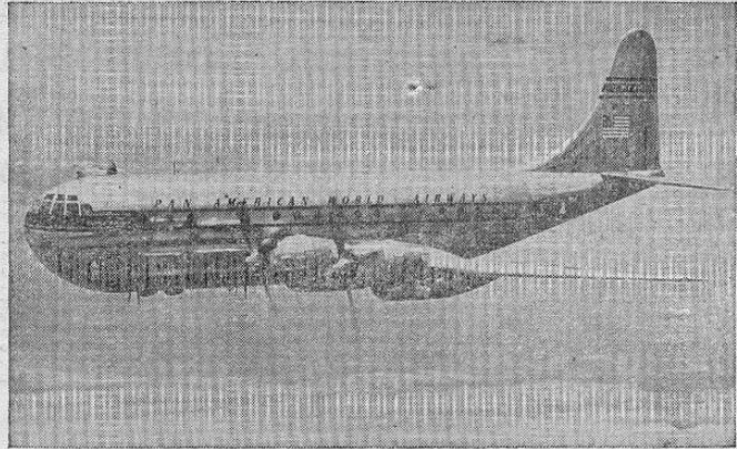
El "América", primero de la flota de veinte clippers tipo Stratecruiser construidos por la Compañía Beeing para la Pan American Airways, y que está acercándose al final de sus vuelos de prueba. Los inmensos cabineros de dos pisos, y cuyo costo asciende a $ 1,500,000, alojarán a 75 pasajeros y contendrán cabinas con camas, como cocinas, un salón y una cantina. Los aviones de 70 toneladas están propulsados por cuatro motores Pratt y Whitney Major de 28 cilindros y 3,500 caballos de fuerza. Cuando entren en operaciones comerciales corrientes, los vuelos desde San Francisco, California, hasta Honolulu, Islas Hawaii, serán reducidos de 12 a 8 y media horas y el vuelo desde Nueva York a Londres se acortará desde 14 y media a 12 horas.
